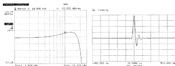
Frequenzgang und Einschwingverhalten des Bezier-Interpolators plus IIR-Filter
