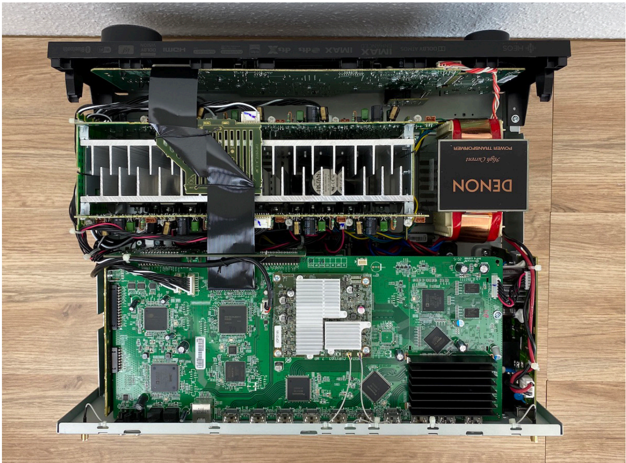
Innerer Aufbau des AVC-X3700H
