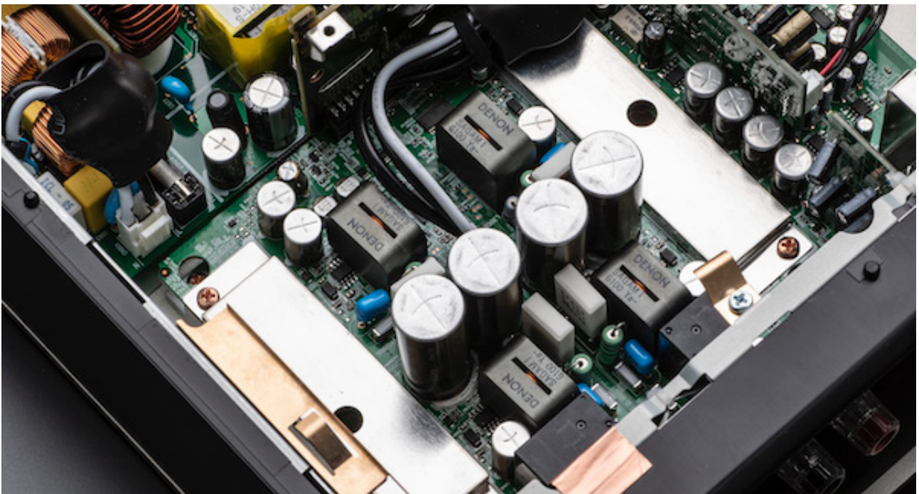
Endstufen-Sektion im PMA-150H
