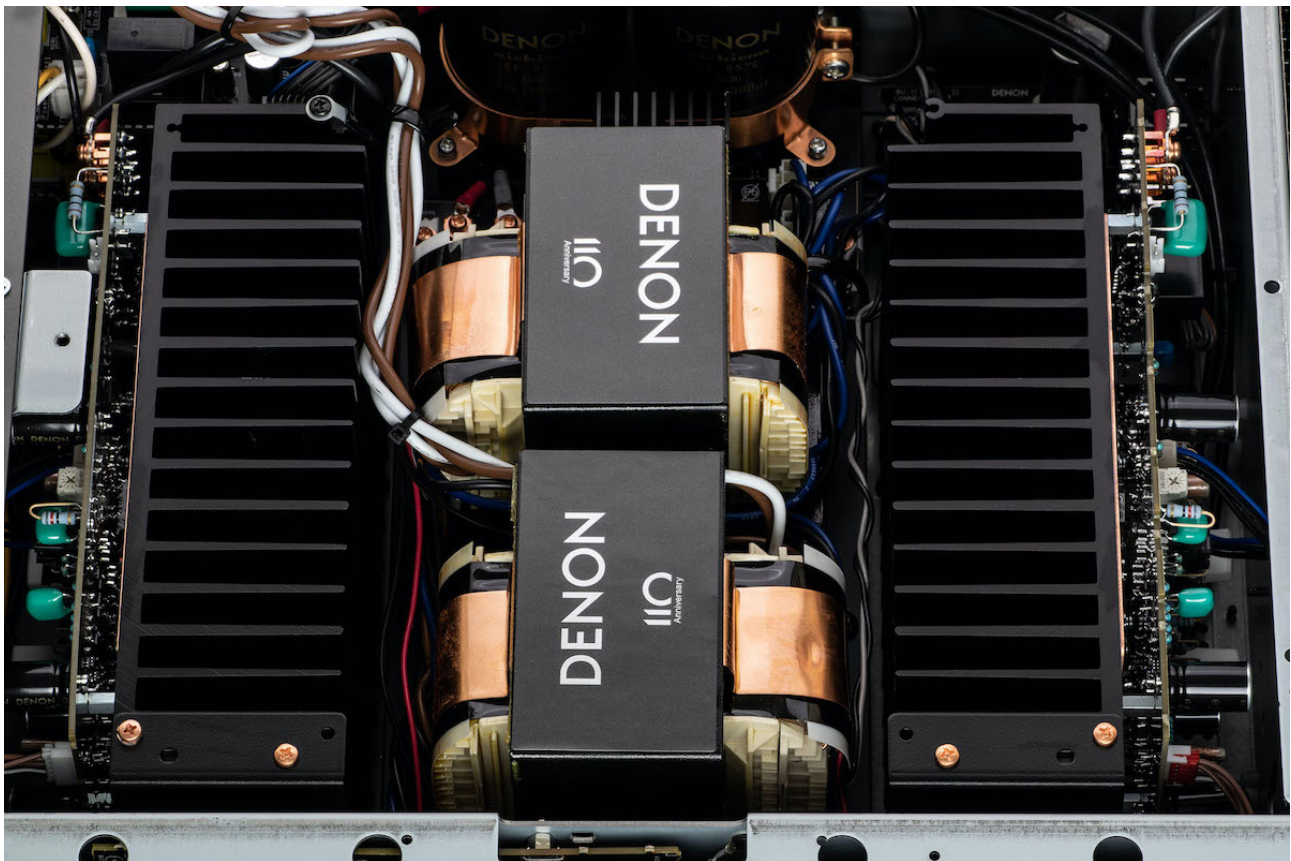
Twin-Transformer im Denon PMA-A110
