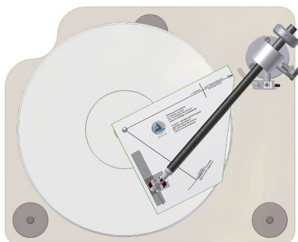
Abb. 10: Absenken des Tonabnehmers auf der Schablone
