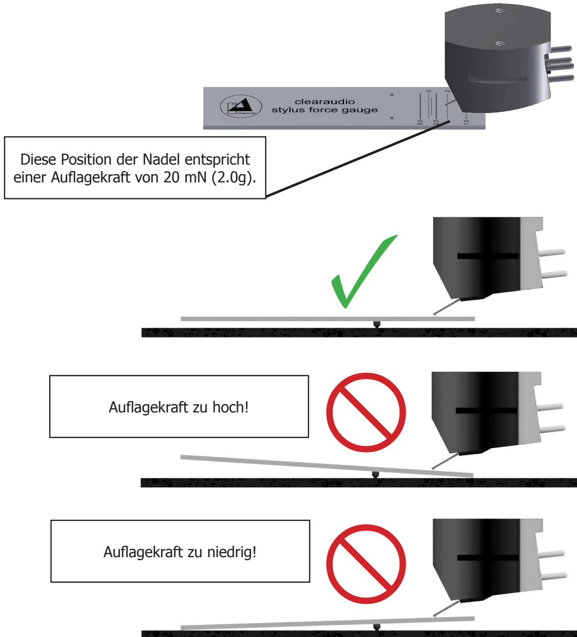
Abb. 8: Einsatz der Smart Stylus Gauge
