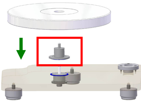
Abb. 3: Aufsetzen des Lageroberteils
