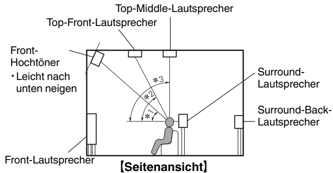
[Seitenansicht]
