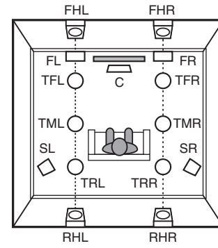
[Draufsicht]
