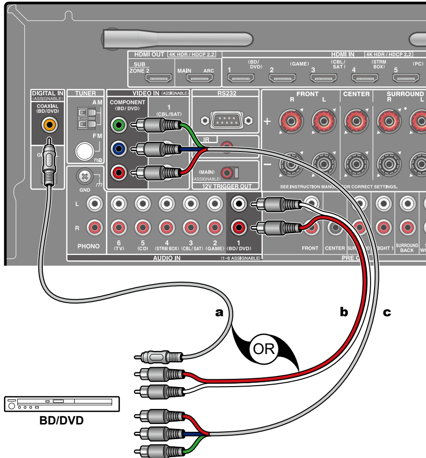
a Digitales Koaxialkabel, b Analoges Audiokabel, c Component-Videokabel
