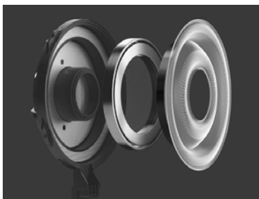
Keunikan: Transduser radiator cincin 56 mm yang paling mutakhir adalah yang terbesar yang pernah digunakan pada headphone.
