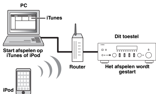
iTunes (voorbeeld)
